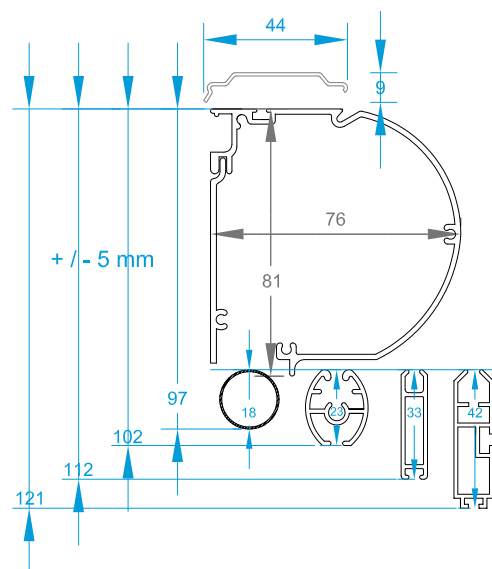
Dimensions des barres de charges compatibles
