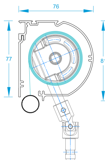
Treuil sortie 45° sous coffre
