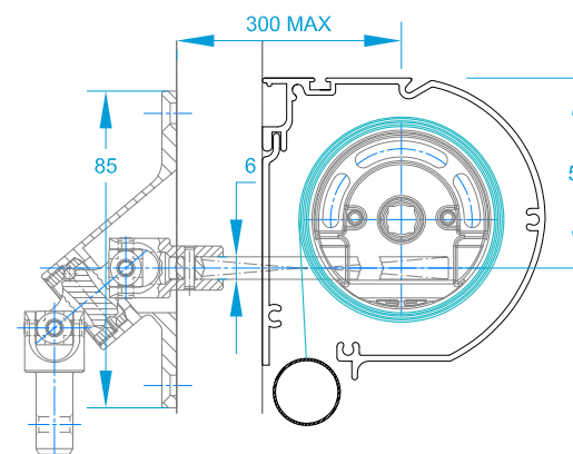
Treuil sortie déportée
