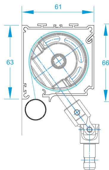
Treuil sortie 45° sous coffre
